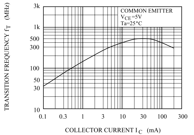
f_T - I_C
