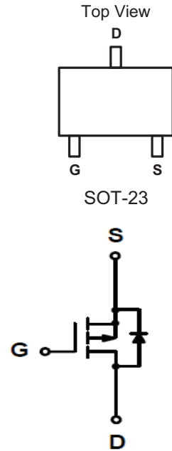
P-Channel MOSFET
