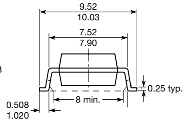
SFH6286 Option
